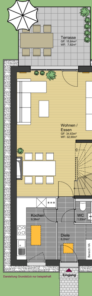
ERDGESCHOSS
